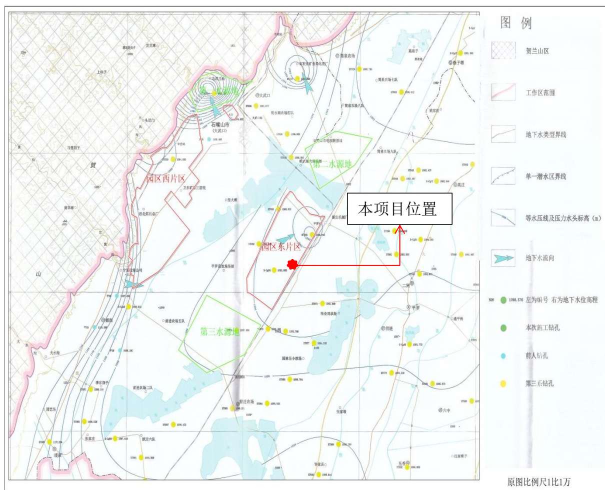
图 3.1-3 项目所在区域地下水流向图
