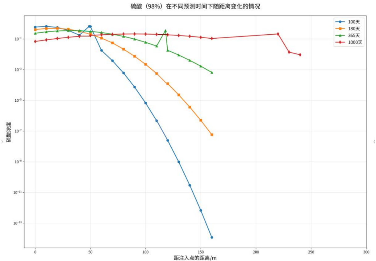
图 6.6-1 硫酸（98%）泄漏对地下水影响分析图
