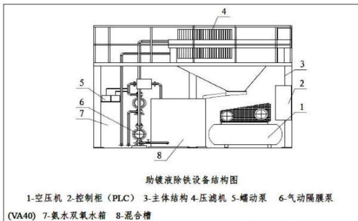
图 5.2-10 废助镀液除铁设备结构示意图
