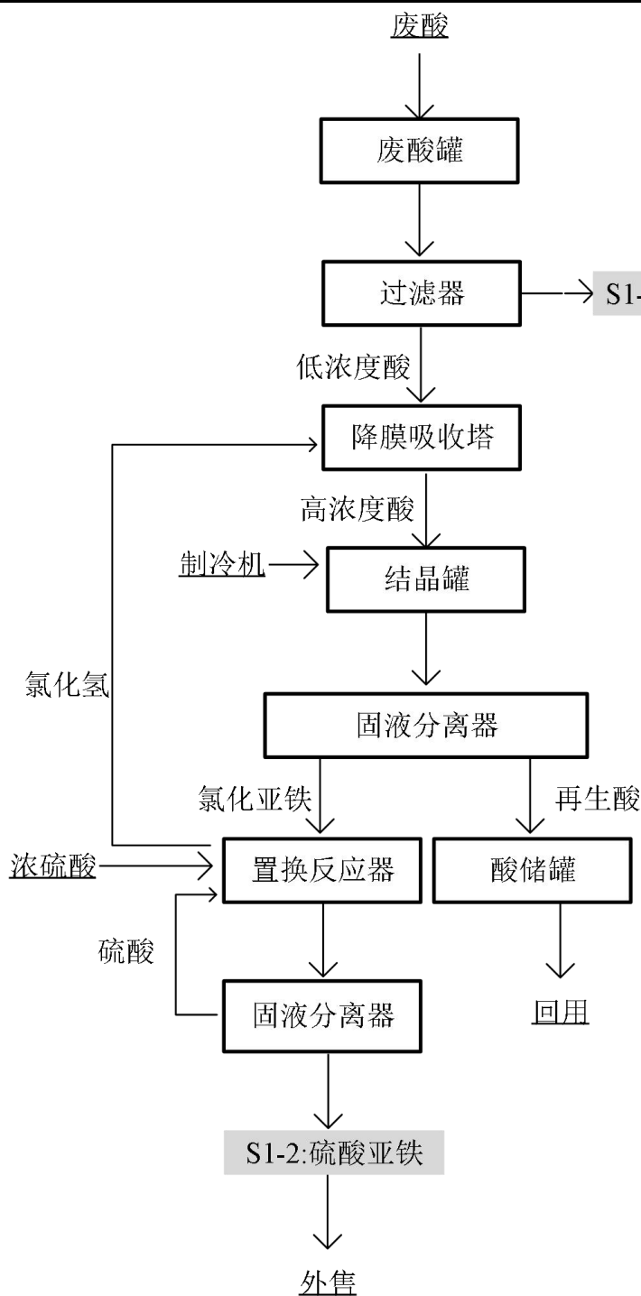
图 2.2-1 废酸再生工艺流程图
