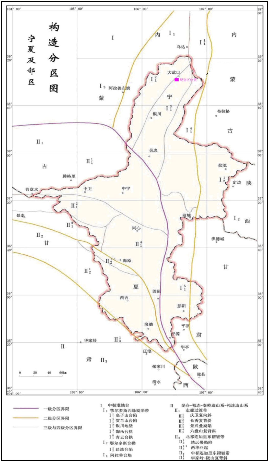
图 3.1-3 宁夏及邻区构造分区图
