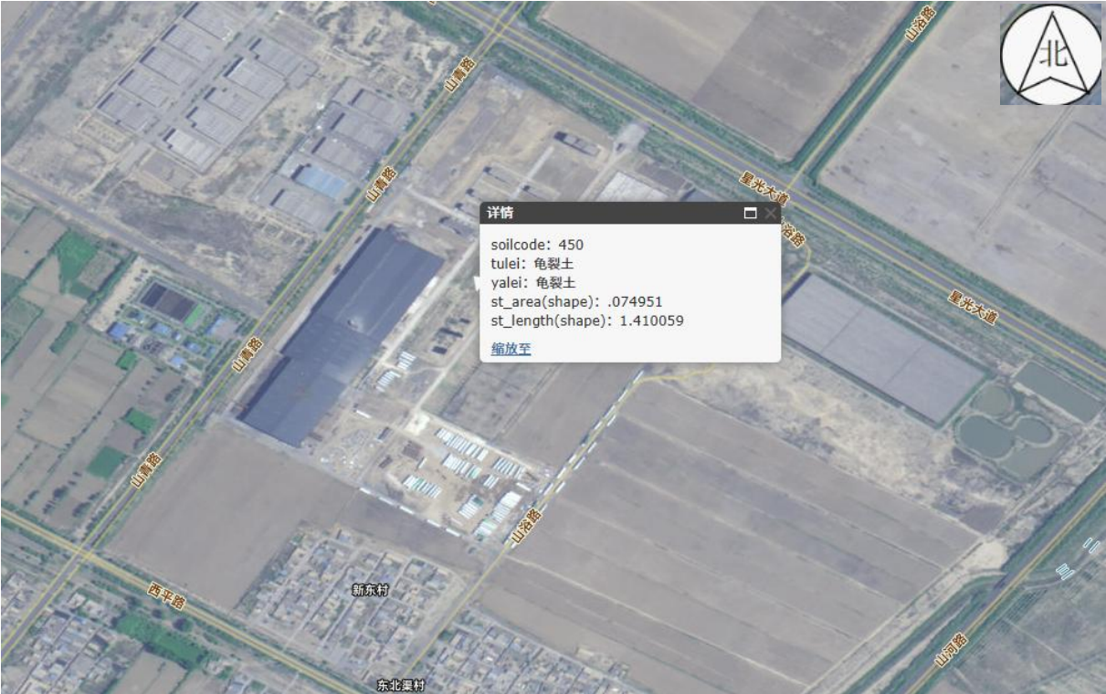
图 3.3-2 项目所在区土壤类型图
